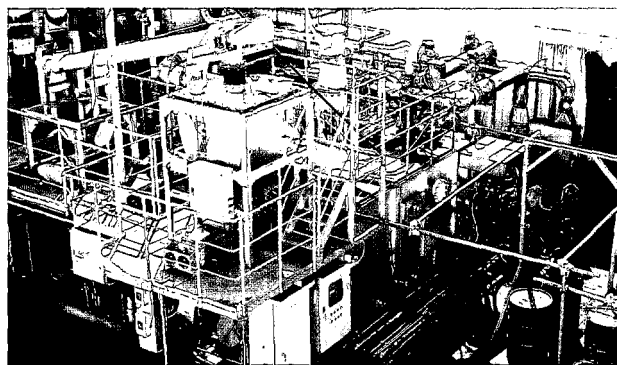
下水污泥から、吸着能力を有した付加価値の高い活性炭化製品を製造することができる「污泥活性炭化設備」
