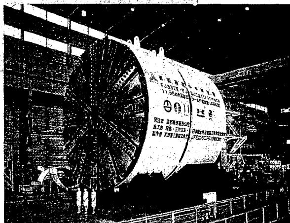
首都高速中央環状新宿線トンネル工事向けシールド掘進機
