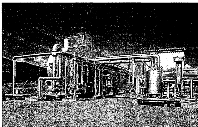
家畜排泄物のメタンによるバイオガス発電設備(北海道・湧別町)
