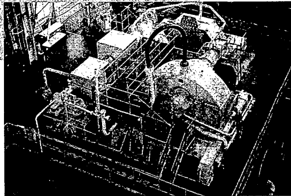
船用蒸気タービンプラント
