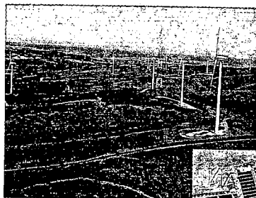
大型風力発電設備
